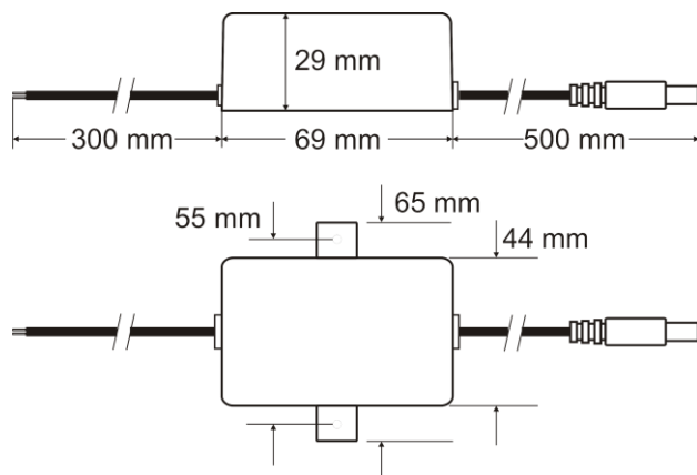
Rys.1. Widok mechaniczny zasilacza.
